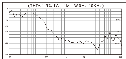
失真特性
