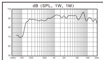
频响特性
